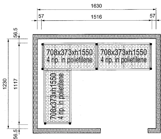
Boven aanzicht
